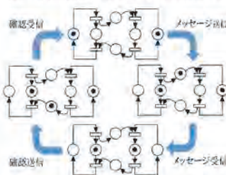
図2 ペトリネットモデルの動作
